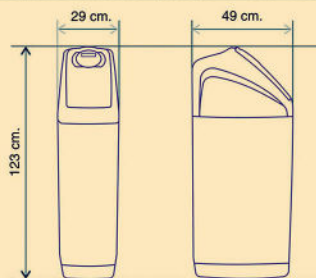
Dimensiones BLACK CLACK - C25 / C38
