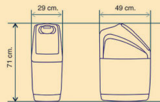
Dimensiones BLACK CLACK - C16
